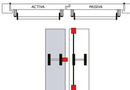
PORTA 2 FOLHAS
