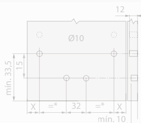
Medidas de furação - Frontal
